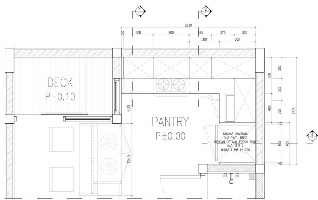
DENAH DAPUR SKALA 1:25
